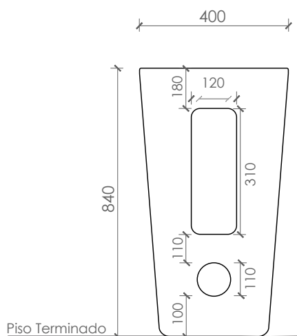
DETALLE POSTERIOR ESC. 1:10
