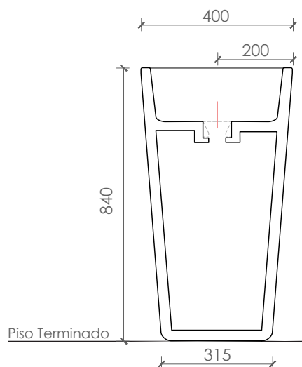
DETALLE FRONTAL ESC. 1:10
